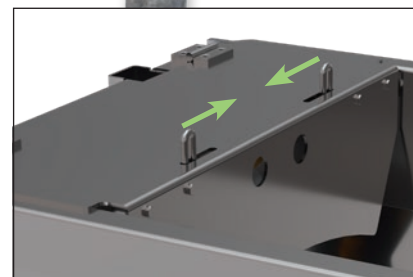
Schwimmer-Abdeckklappe mit Schnellverschluss
